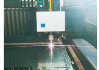
切断加工作業
